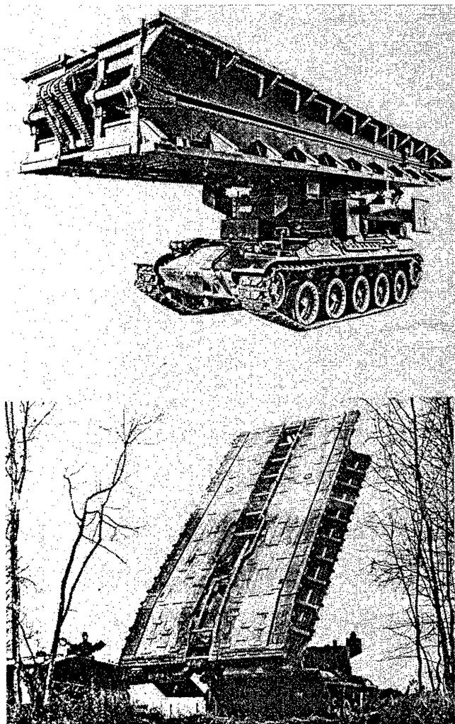
Slika 5. Francusko vozilo guseničar AMX-30 sa mostom dvodelne konstrukcije
